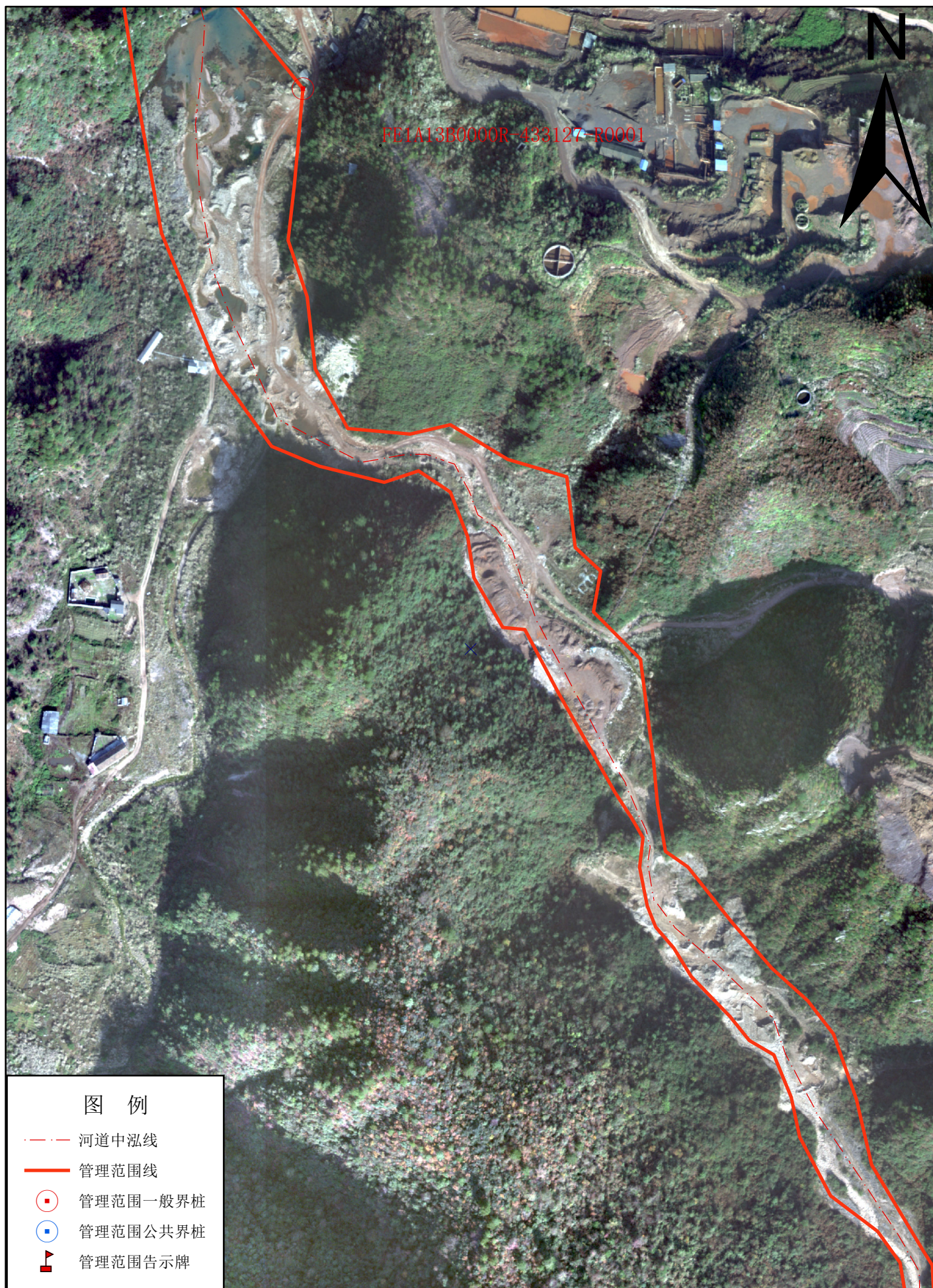
桃子溪河湘西自治州永顺县河段管理范围划定图（七）
