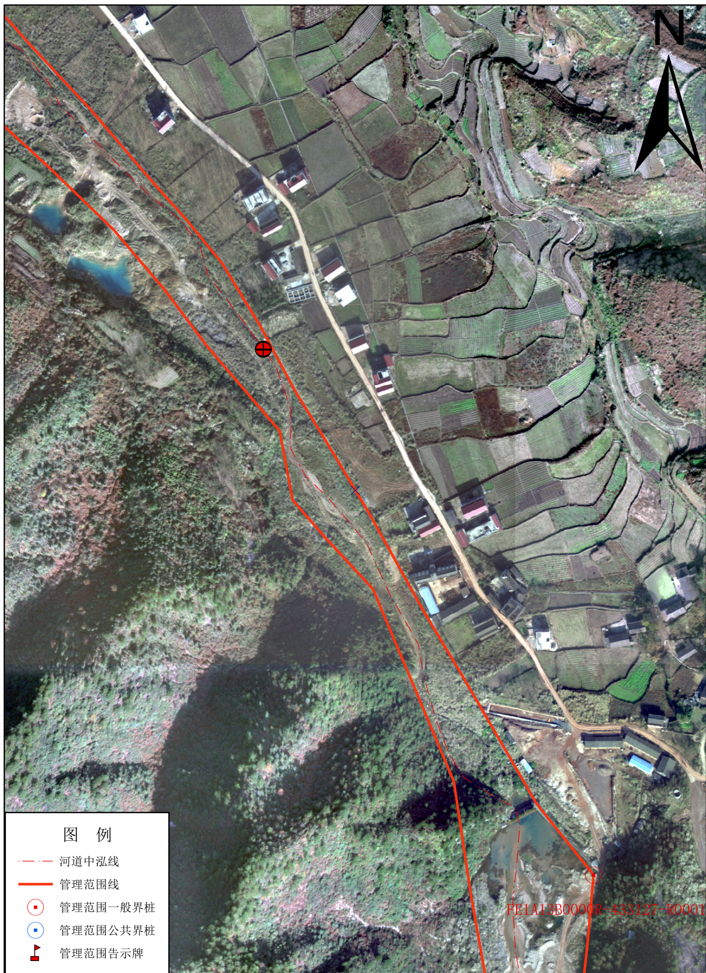
桃子溪河湘西自治州永顺县河段管理范围划定图（六）
