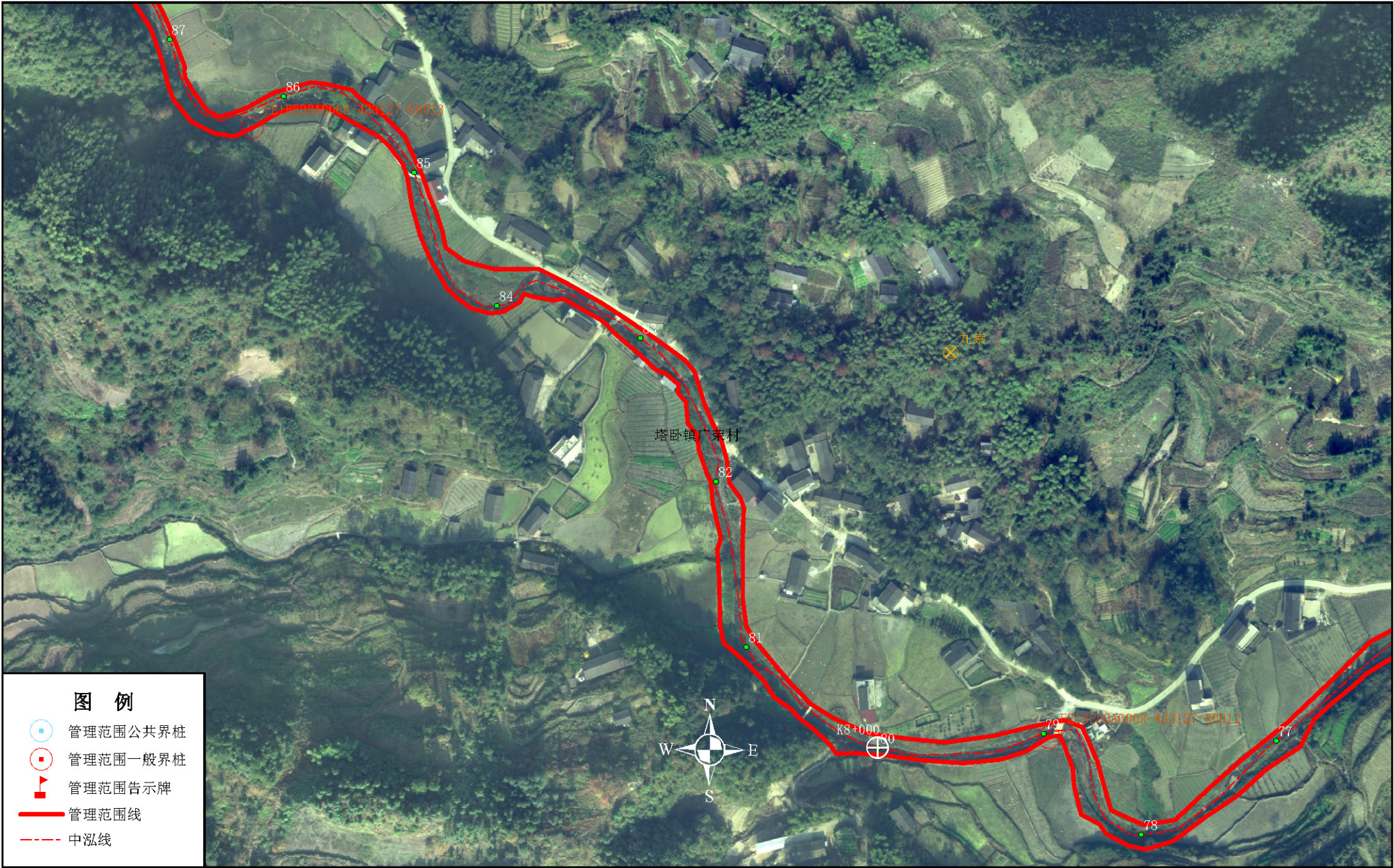
灵溪河永顺河段河道管理范围划定图
